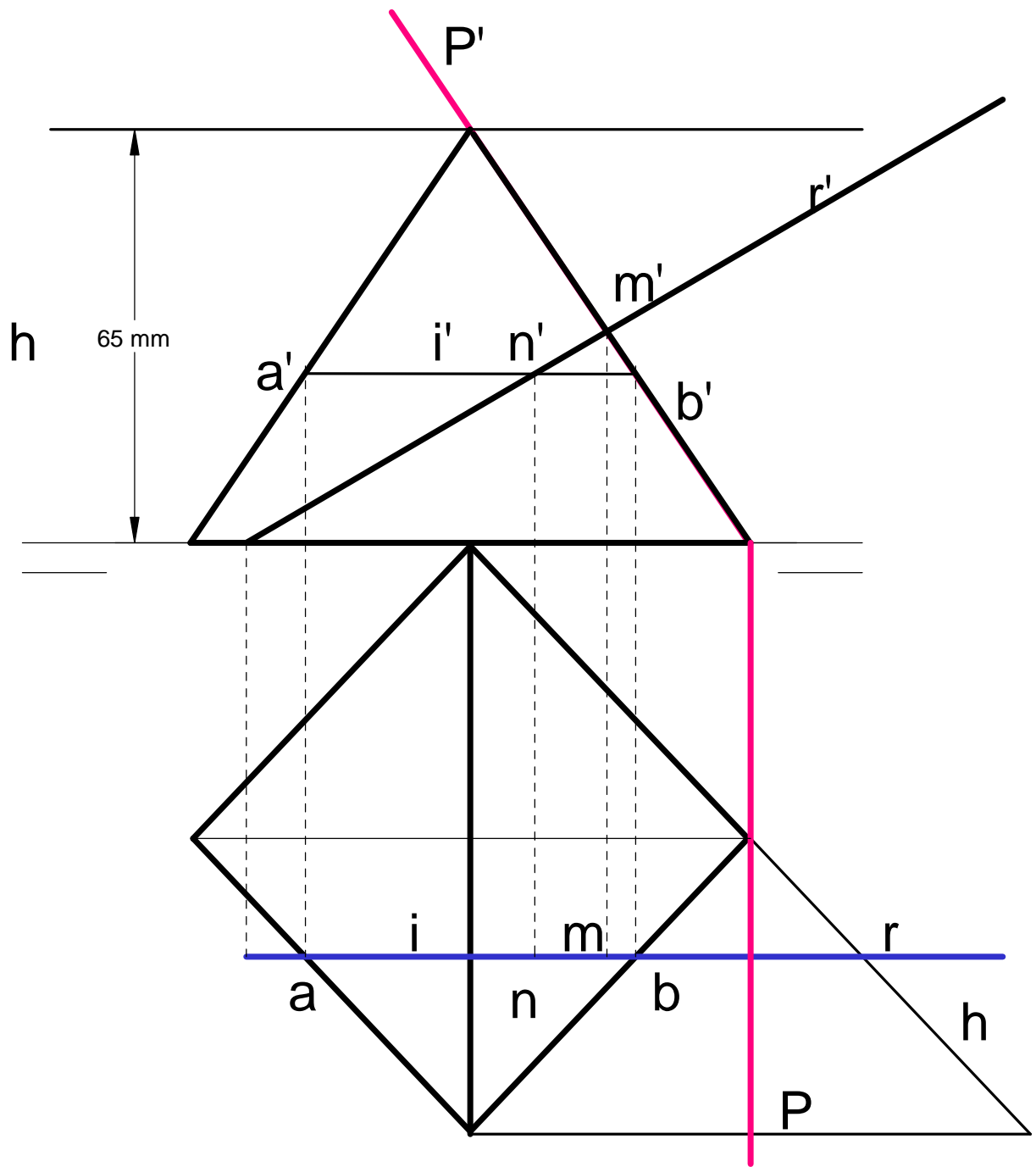
INTERSECCIÓN DE UNA RECTA FRONTAL (R) CON UN TETRAEDRO APOYADO SOBRE UNA ARISTA
